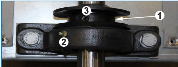
Sluitringsamenbouw
