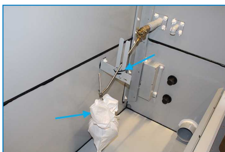
Fastsättning och lindning av flottörkula
