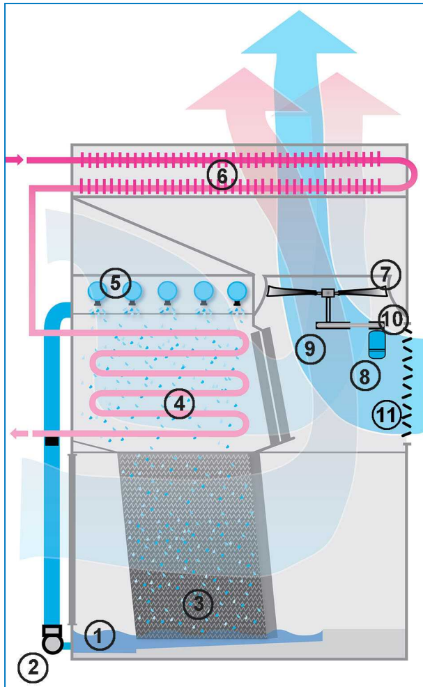
Principe de fonctionnement - Registres de modulation d'entrée d'air ouvert
