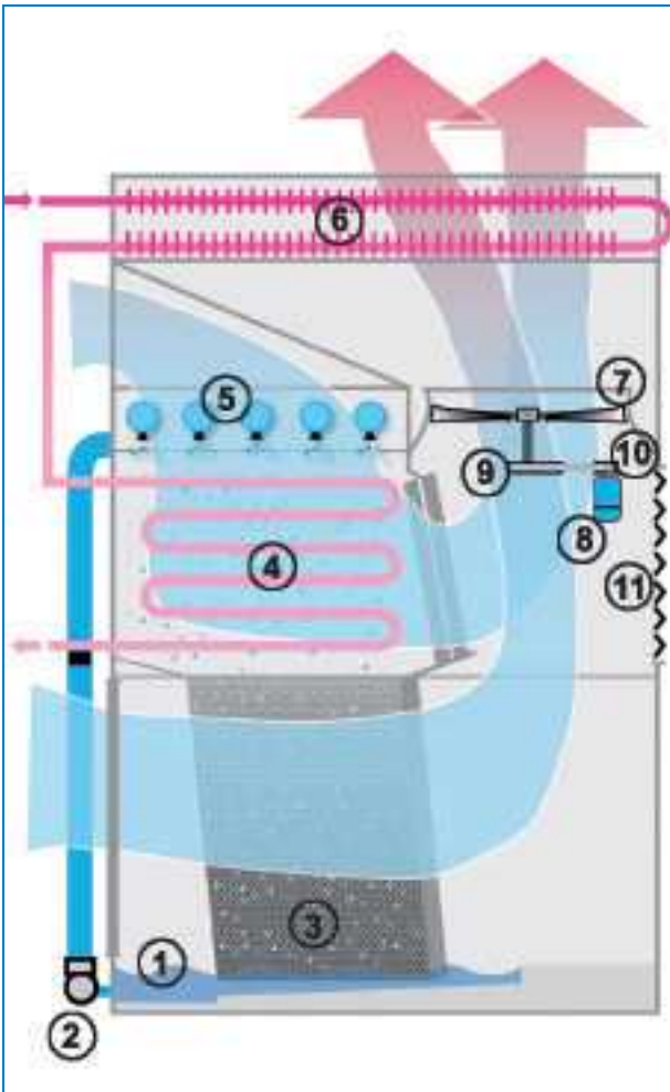
Principe de fonctionnement - Registres de modulation d'entrée d'air
