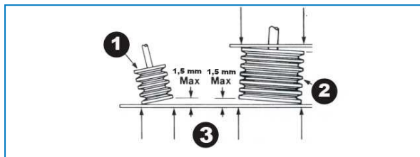
Allineamento delle pulegge nelle trasmissioni standard
