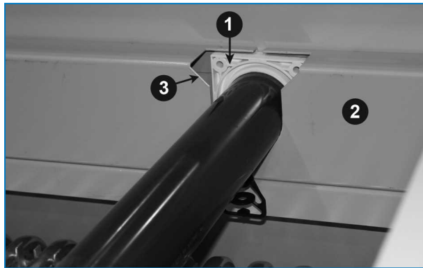
Sistema di spruzzo rimovibile BranchLok™
