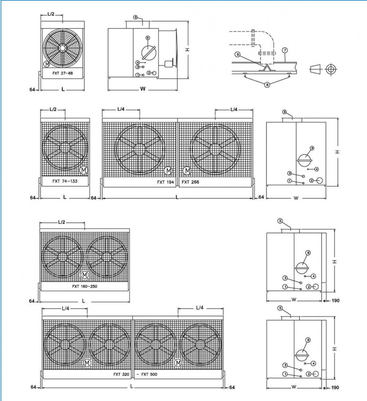
1. Vaciado; 2. Salida agua; 3. Rebosadero; 4. Llenado; 5. Entrada agua; 6. Puerta de acceso; 7. Caja de distribución superior; 8. Orificios calibrados; 9. Divisor de caudal; * Sección de rejilla externa solo en FXT 211, 250, 422, 500.
